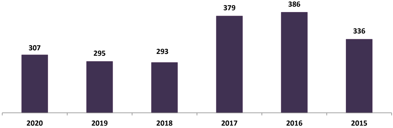
تطور سعر السكر الخام (دولار للطن)
